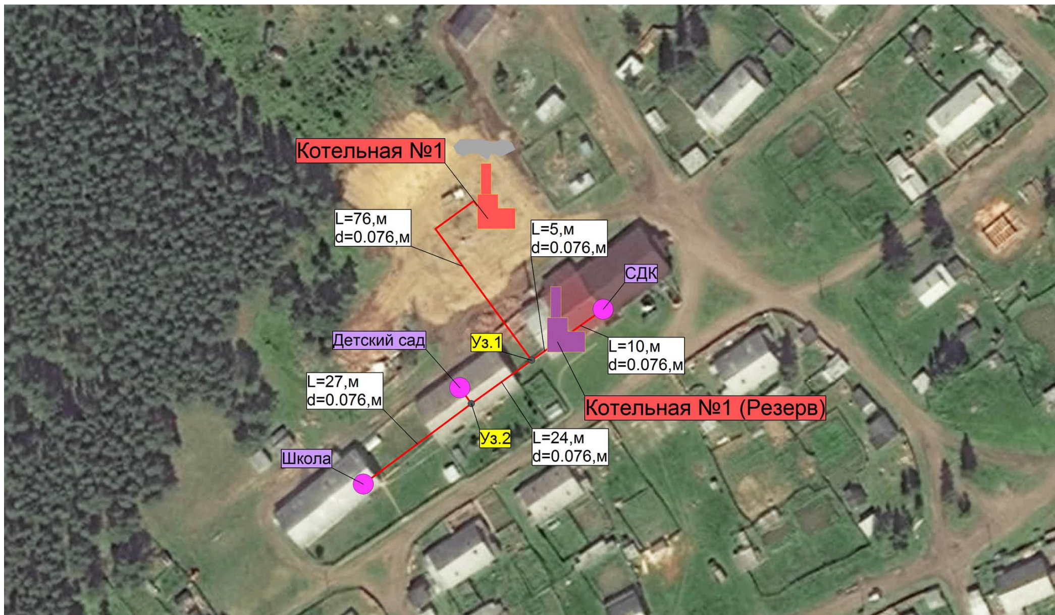
Рис. 2.1.3 – Схема теплоснабжения муниципального образования «Аимское сельское поселение» от котельной №1
