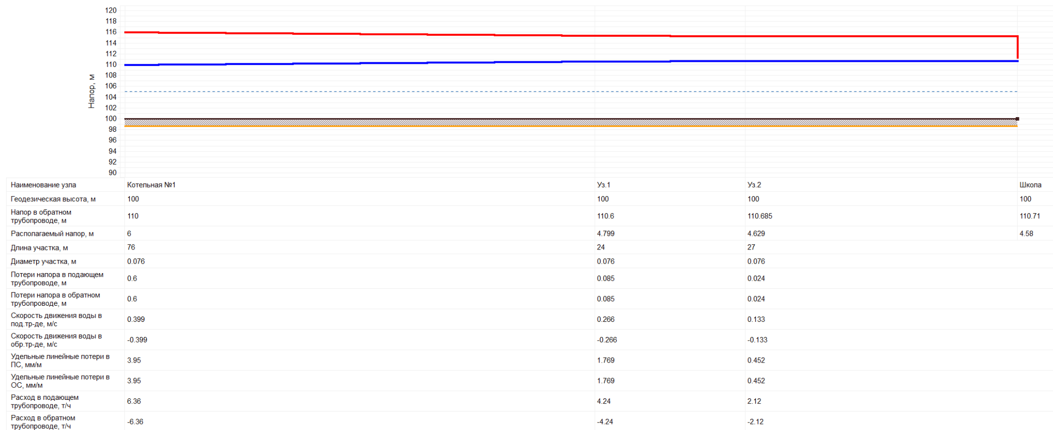
Рис. 2.1.4 – Пьезометрический график от котельной №1 до школы.
