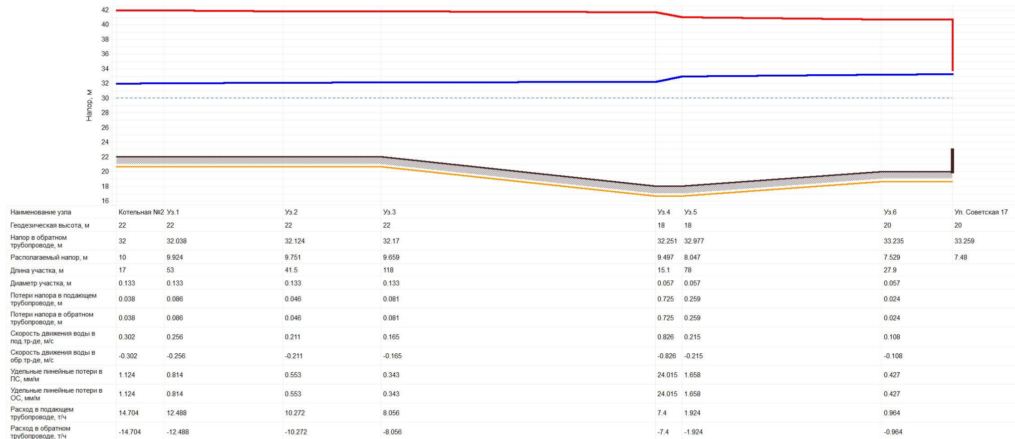
Рис. 2.1.5 – Пьезометрический график от котельной №2 «Школьная» до ул. Советская 17.
