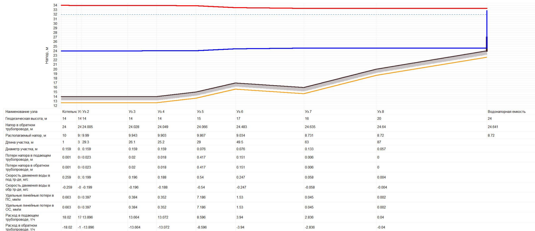
Рис. 2.1.4 – Пьезометрический график от котельной №1 «Центральная» до водонапорной емкости.
