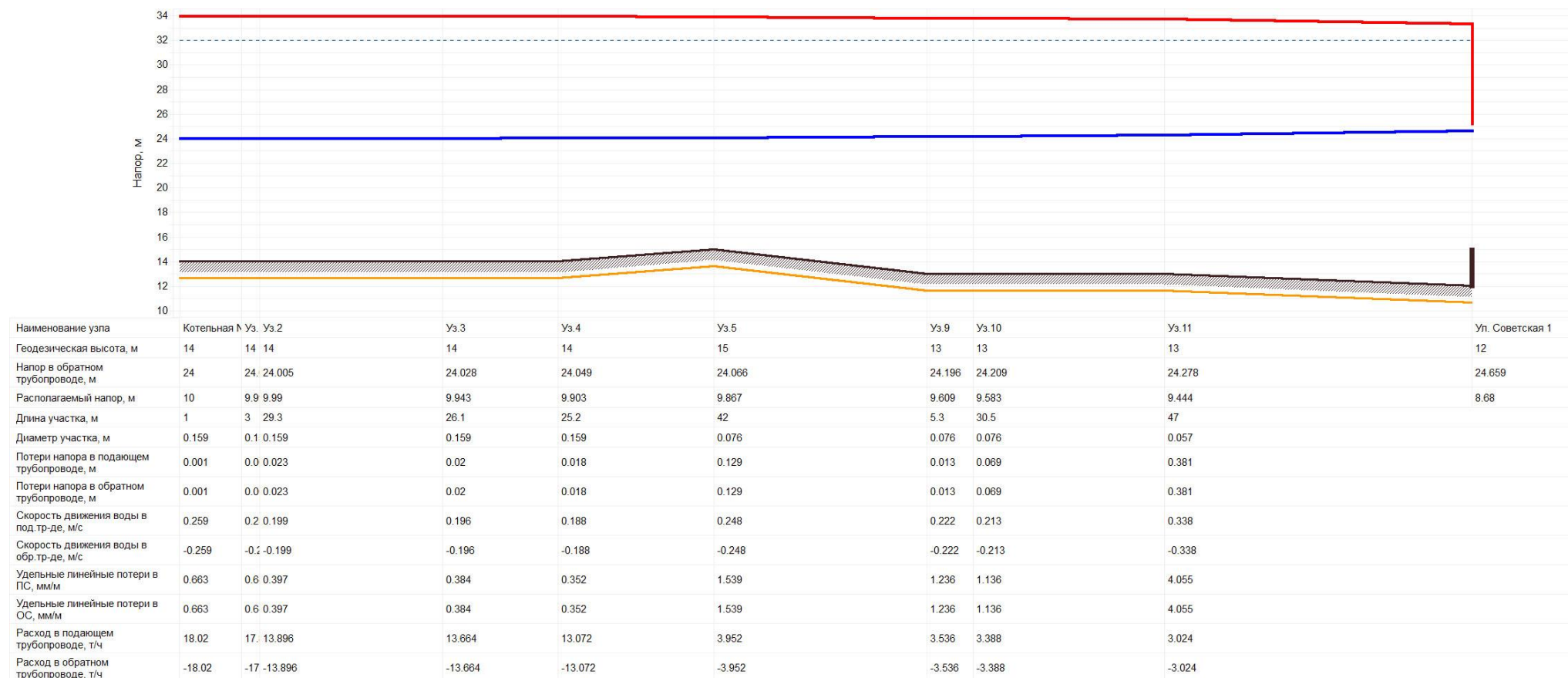
Рис. 2.1.3 – Пьезометрический график от котельной №1 «Центральная» до ул. Советская 1.
