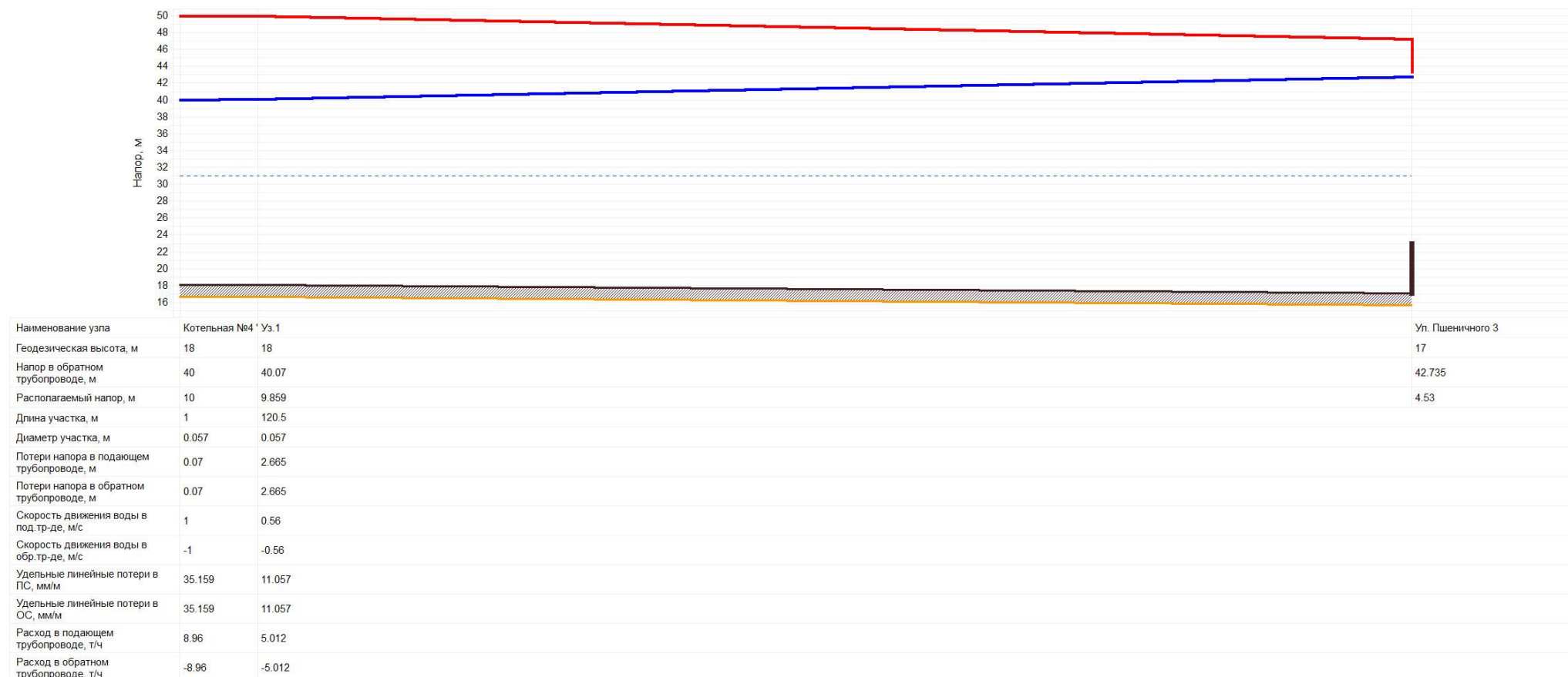
Рис. 1.8 – Пьезометрический график от котельной №4 «Колхозная» до ул. Пшеничного 3.
