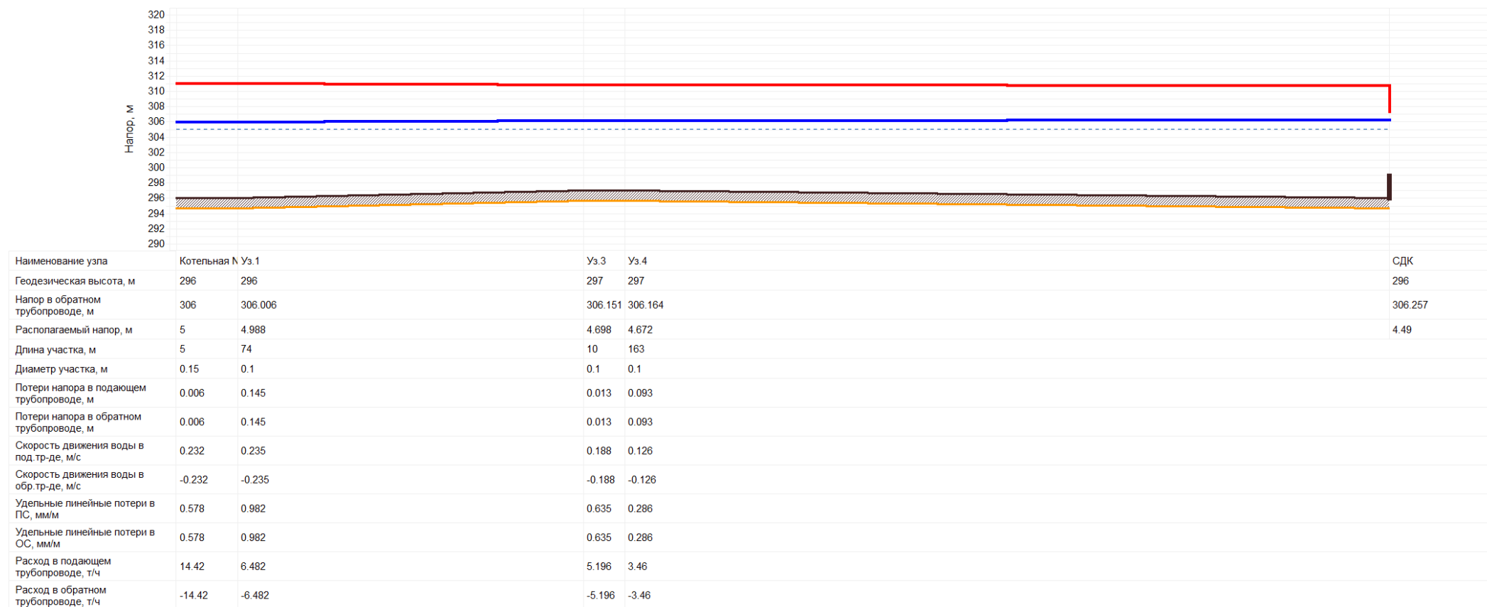
Рис. 2.1.5 – Пьезометрический график от котельной №1 до СДК.
