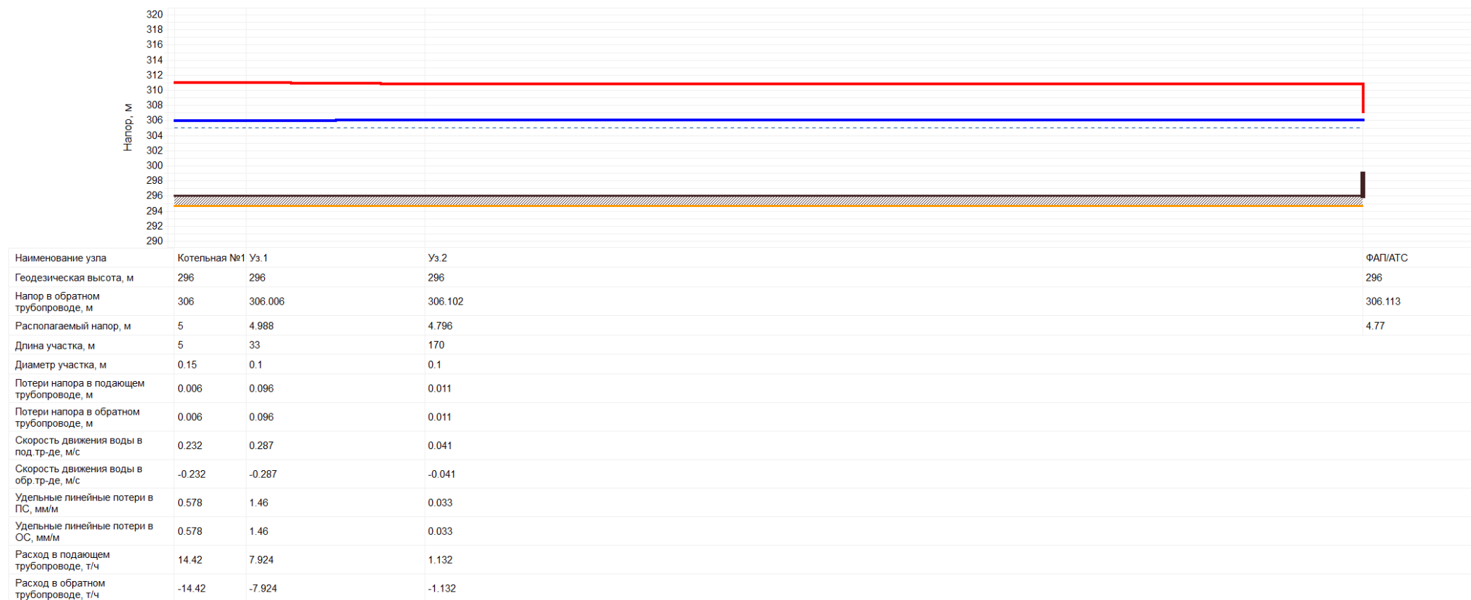
Рис. 2.1.6 – Пьезометрический график от котельной №1 до ФАП/АТС.
