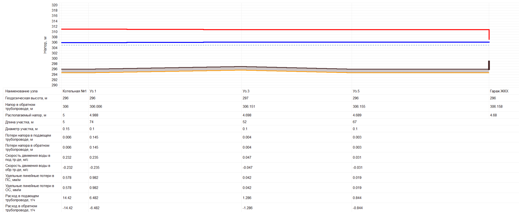
Рис. 2.1.4 – Пьезометрический график от котельной №1 до гаража ЖКХ.
