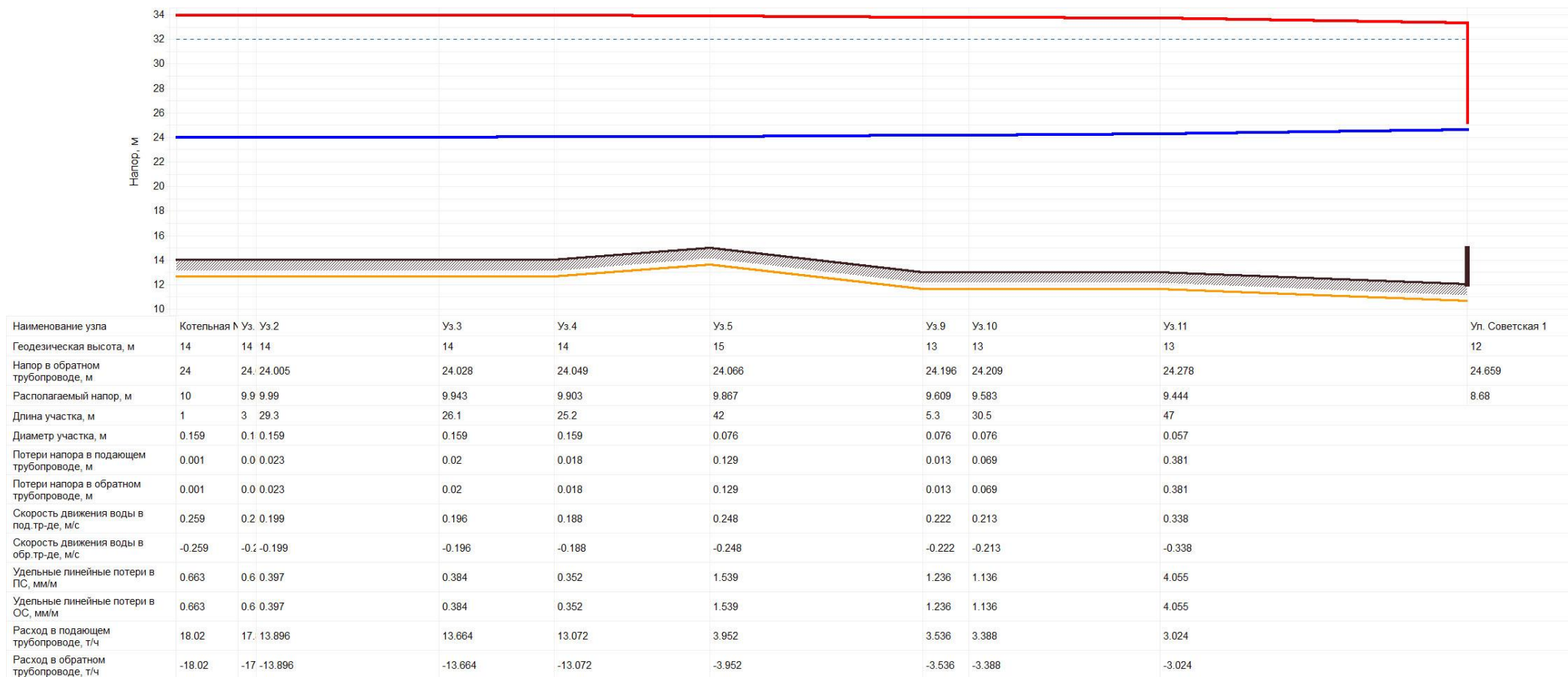
Рис. 1.3 – Пьезометрический график от котельной №1 «Центральная» до ул. Советская 1.
