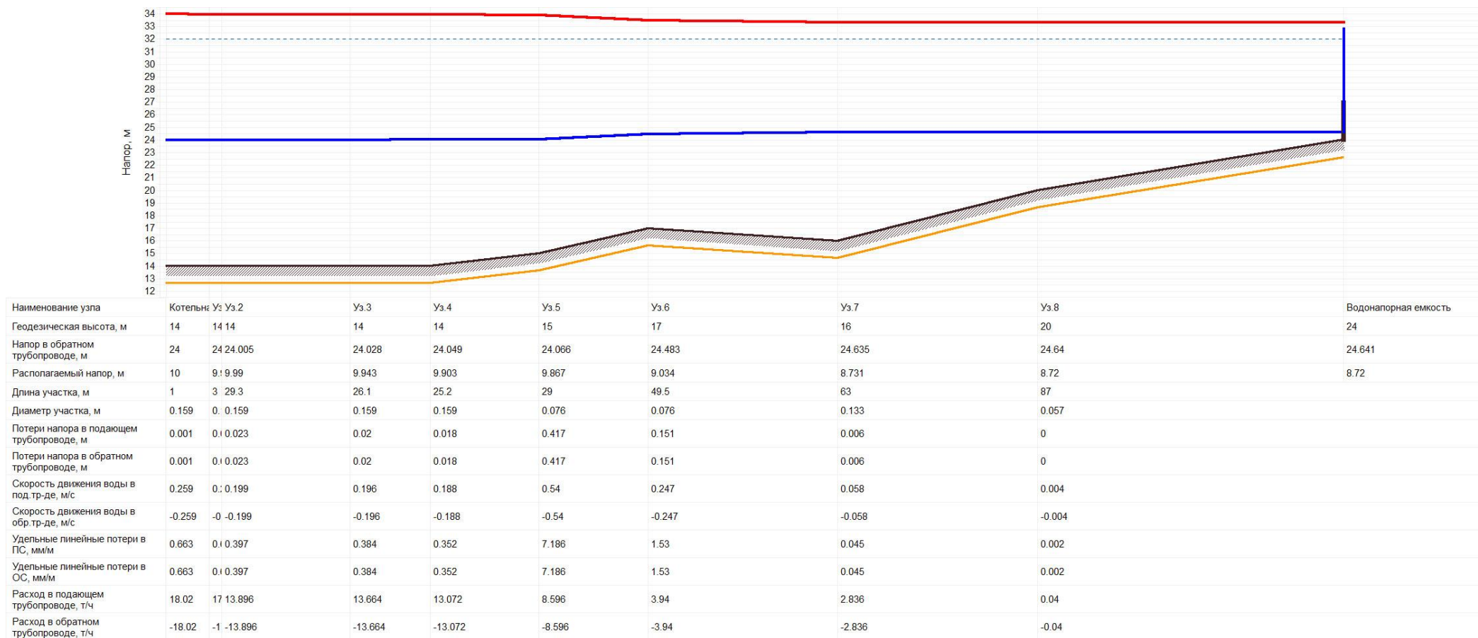
Рис. 1.4 – Пьезометрический график от котельной №1 «Центральная» до водонапорной емкости.
