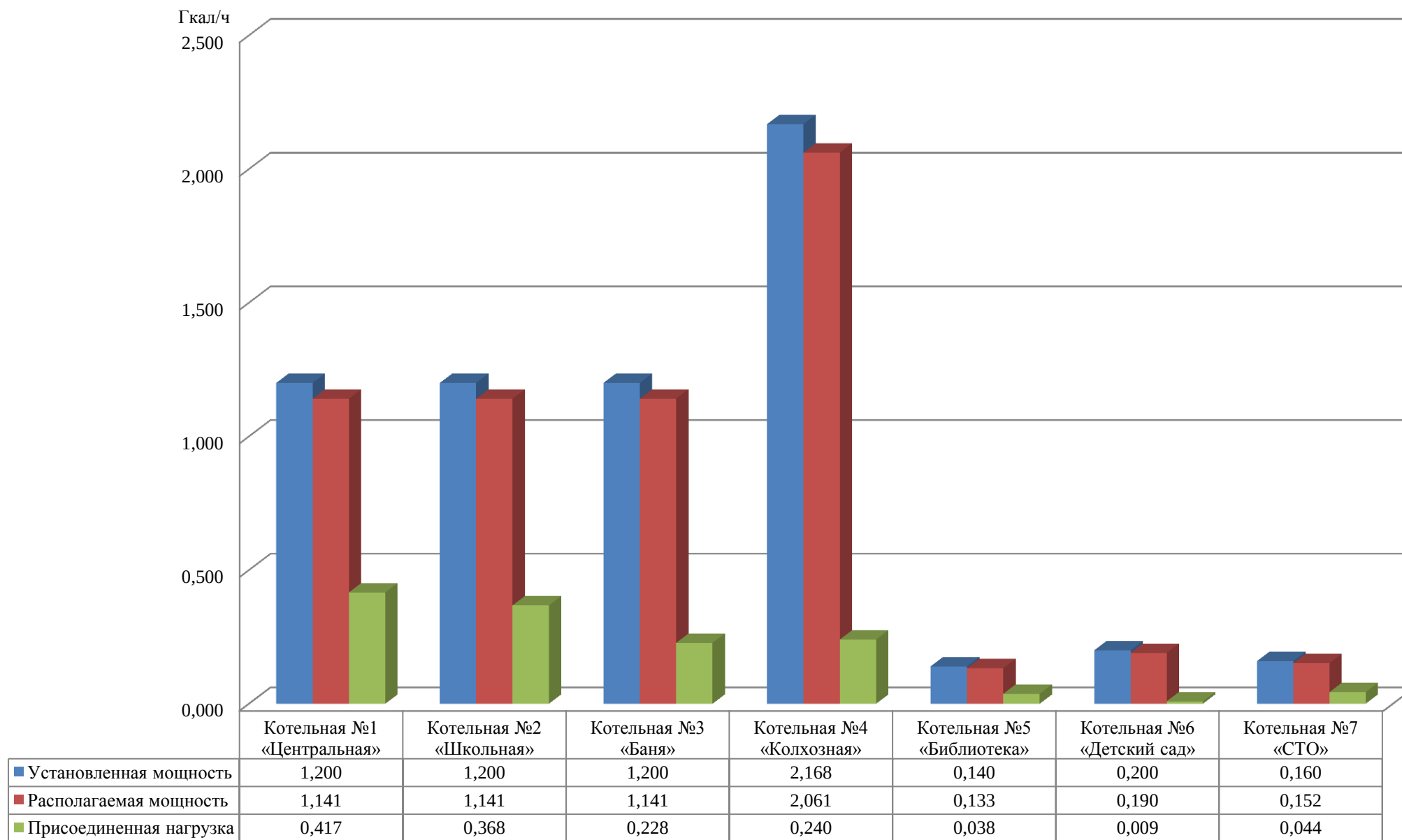
Рис. 1.2 – Распределение мощностей источника тепловой энергии
