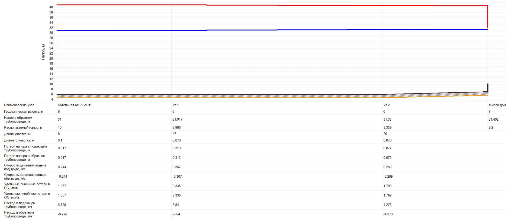
Рис. 1.6 – Пьезометрический график от котельной №3 «Баня» до жилого дома.
