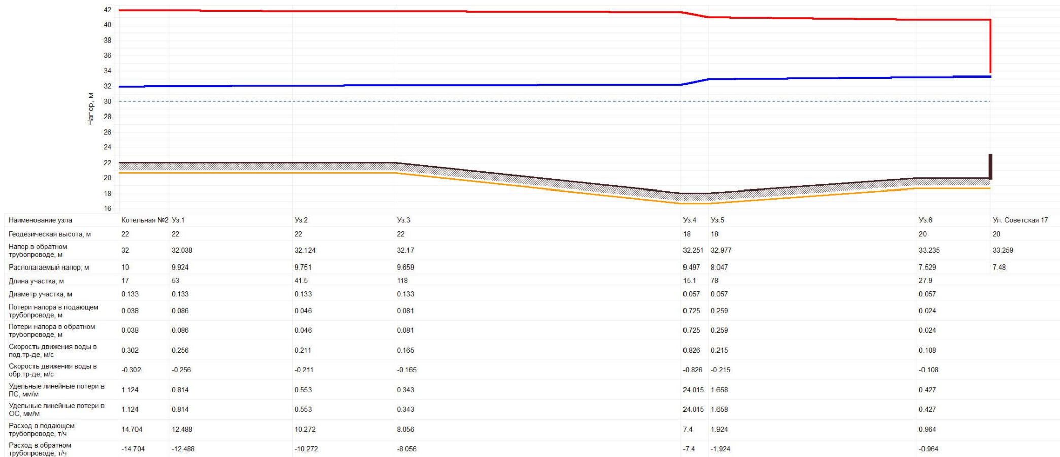
Рис. 1.5 – Пьезометрический график от котельной №2 «Школьная» до ул. Советская 17.
