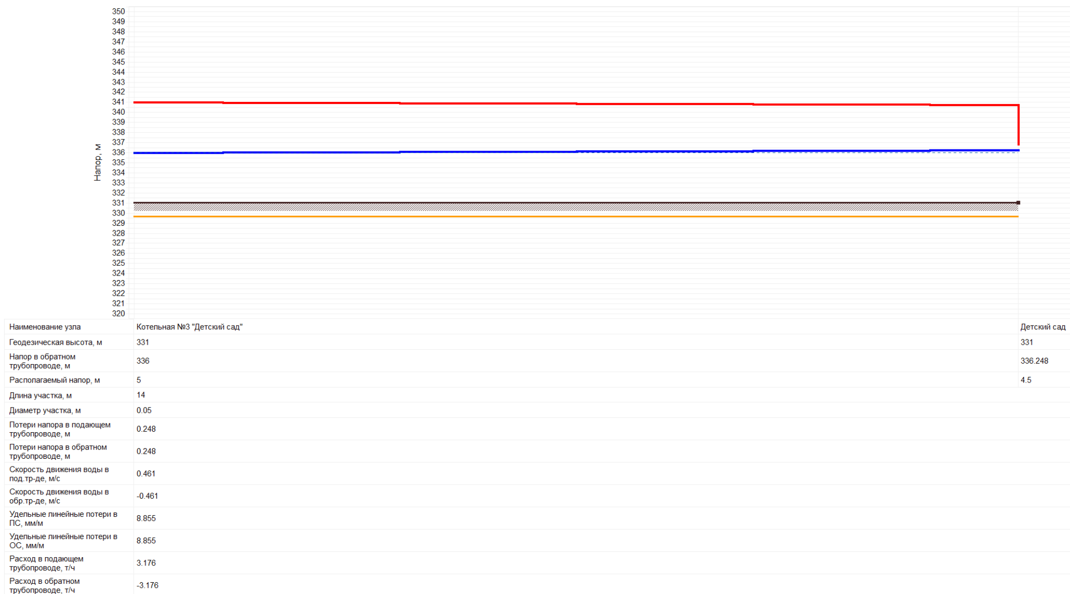
Рис. 1.5 – Пьезометрический график от котельной №3 «Детский сад» до детского сада.
