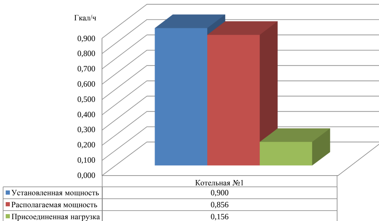
Рис. 1.2 – Распределение мощностей источника тепловой энергии
