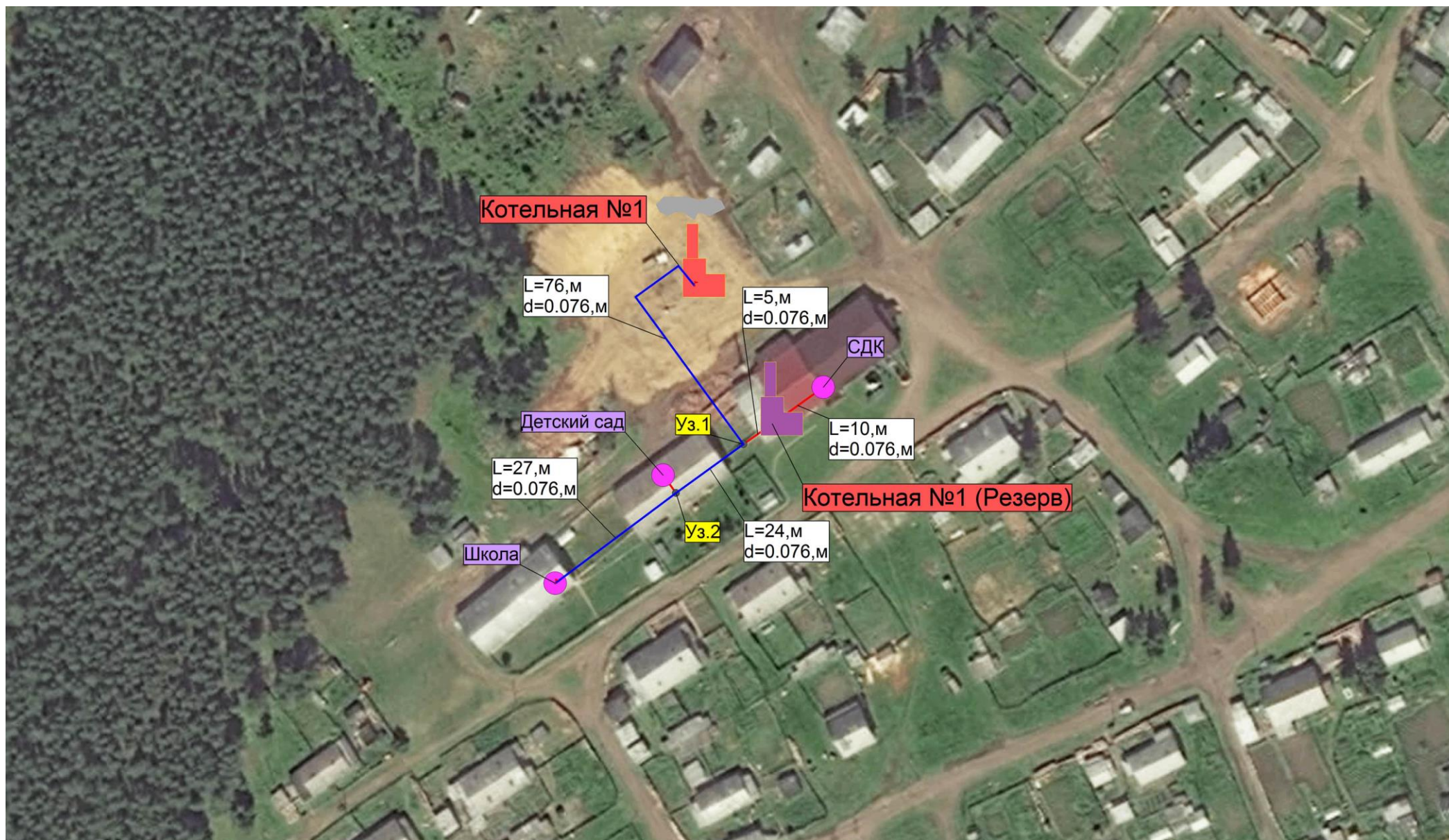
Рис. 8.2 – Расчетный участок тепловой сети
