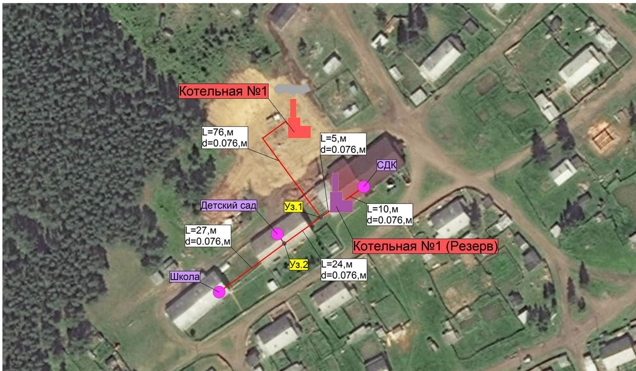
Рис. 1.3 – Схема теплоснабжения муниципального образования «Аимское сельское поселение» от котельной №1
