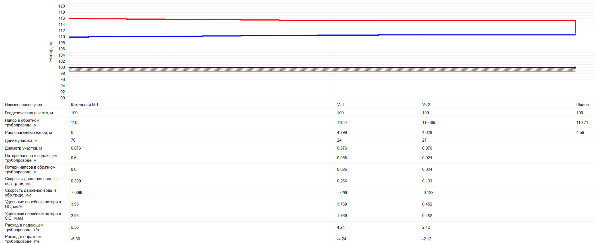
Рис. 1.4 – Пьезометрический график от котельной №1 до школы.
